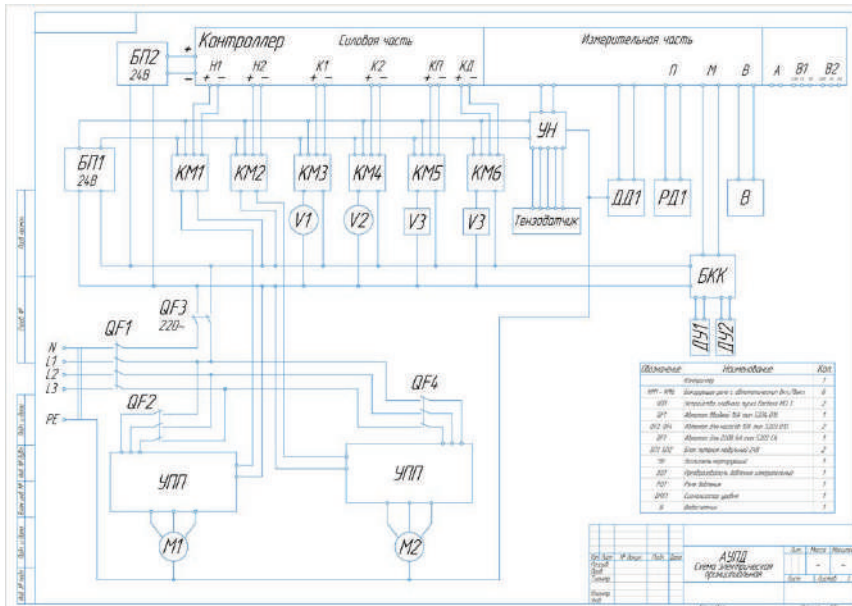
Рис.3 Электрическая принципиальная схема
