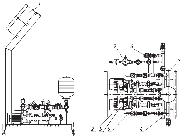
Рис.1 Состав установки Westermat 2CM3-8
